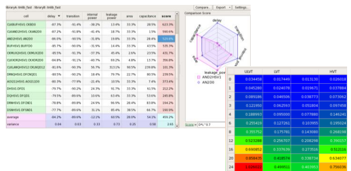
标准单元的PPA性能比较及趋势分析结果
